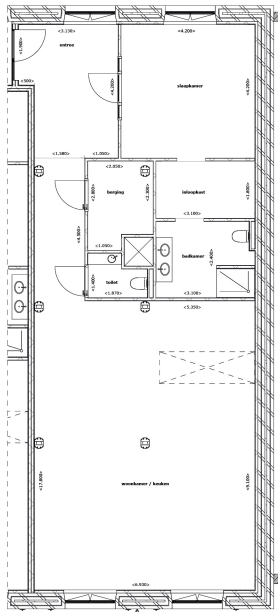
Plattegrond verdieping 02 1:50
